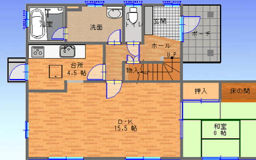
1階平面図
